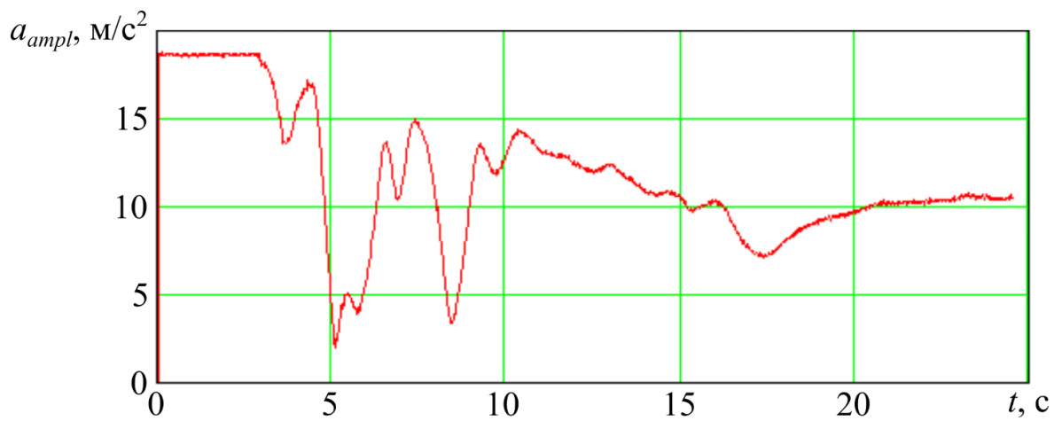
Рисунок 4.18 – Зміна амплітуди вібраційного прискорення при русі преса віброгасника вниз
