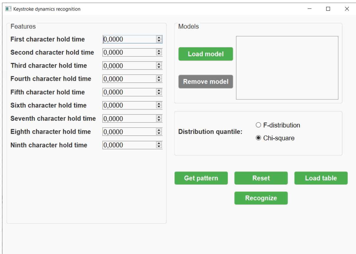
Рисунок 4.3 – Графічне вікно застосунку для розпізнавання клавіатурного почерку
