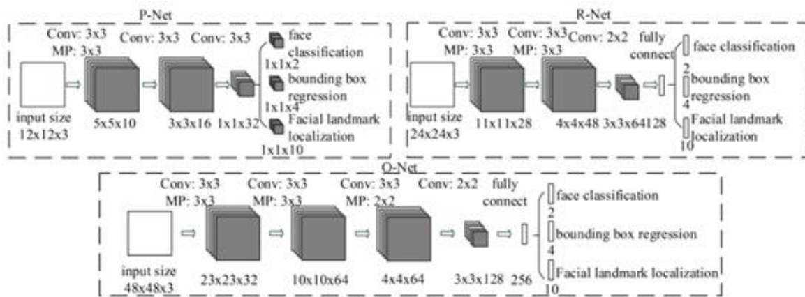
Рисунок 1.4 – Структура MTCNN [85]
