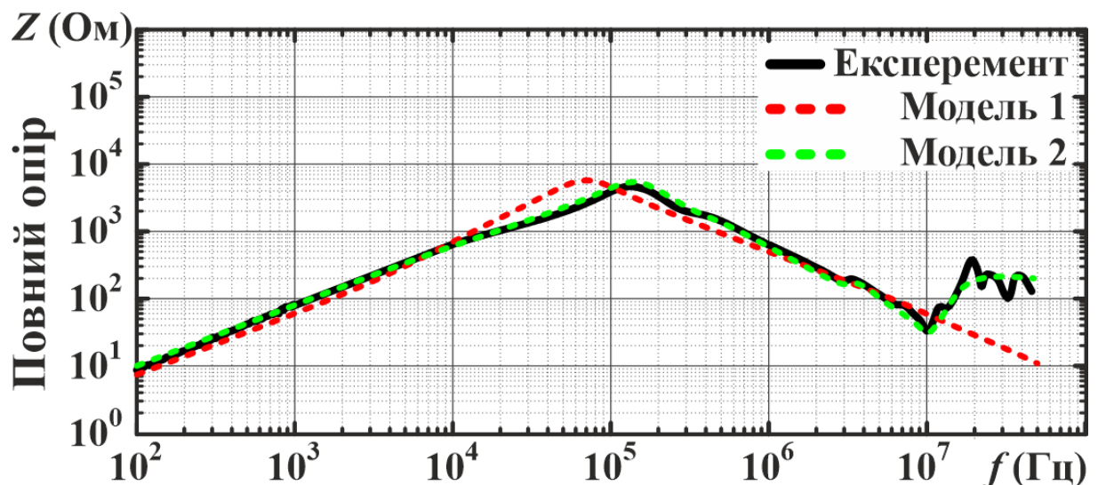
Рисунок 2.9 – Частотні залежності повного опору в синфазному(а) та диференційному режимах (б) отримані експериментально та за рахунок числового моделювання
