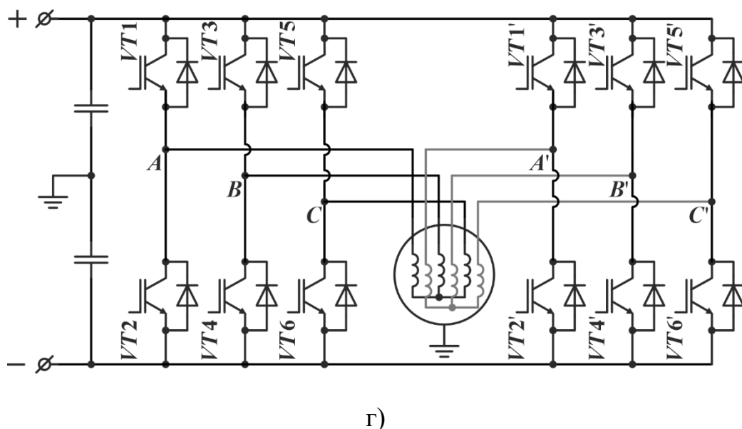
Рисунок 3.4 – Схеми модифікованих топологій інвертора та машин:
