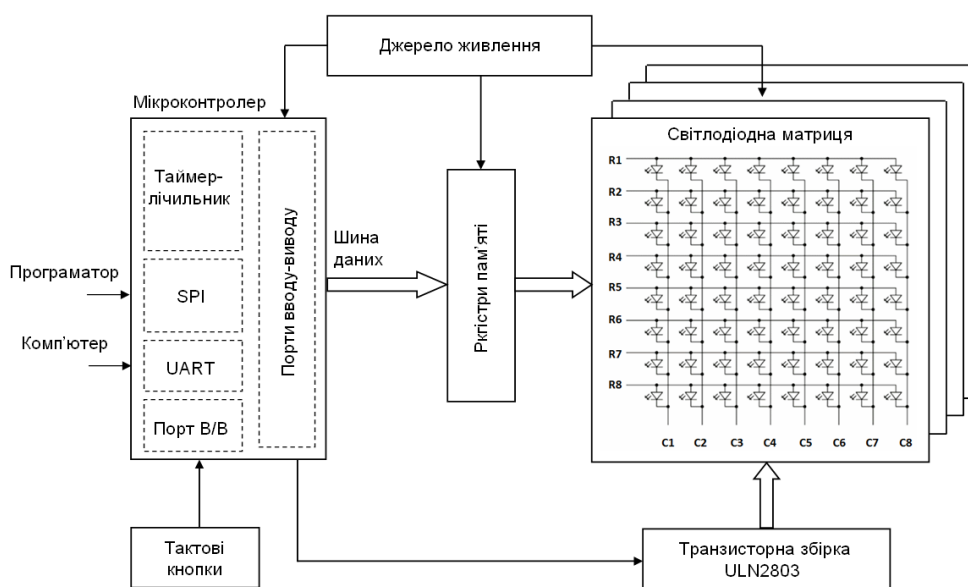
Рисунок 1.5 – Структурна схема мікропроцесорної системи відображення інформації
