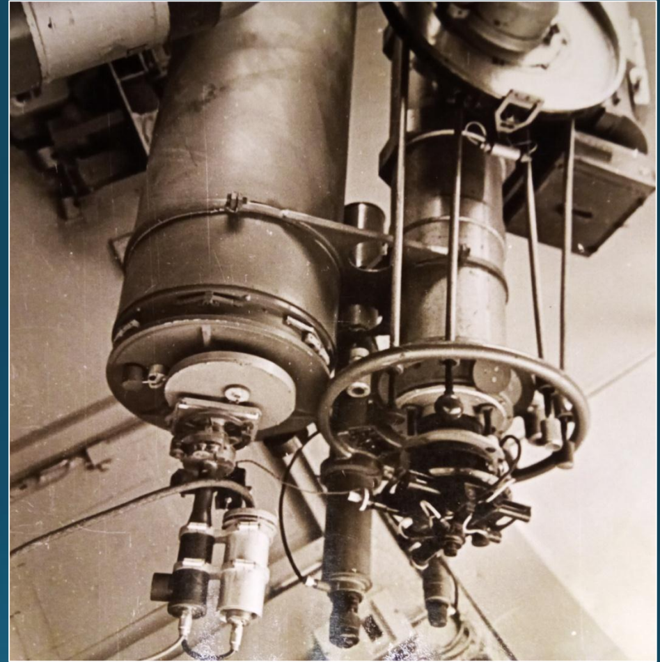
200 мм телескоп разом з 400 мм телескопом- рефлектором
